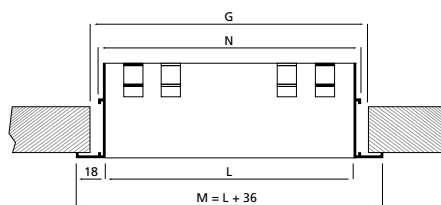
Coupe longitudinale du diffuseur seul
