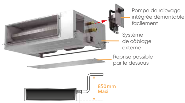
Accessoire de raccordement des condensats fourni de série.
