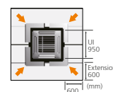
Extension de façade UTG-AGYA-W
